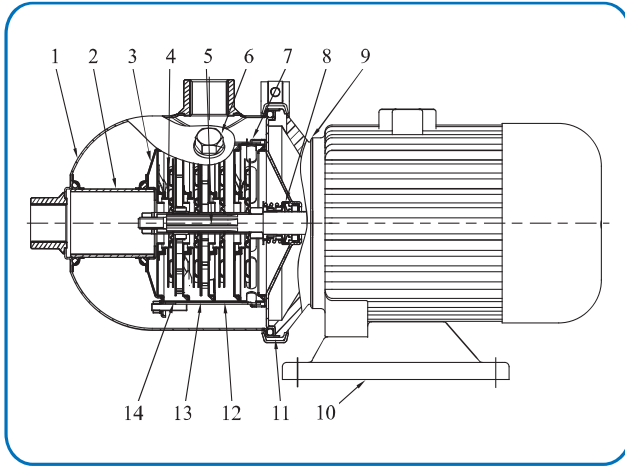
截面图 CHL, CHLK2,4
