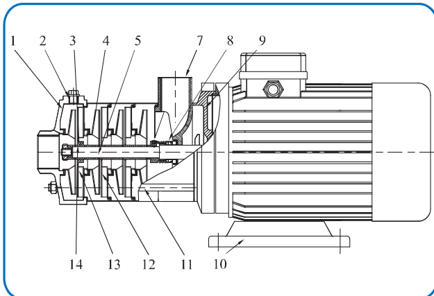
截面图 CHLF, CHLF(T)
